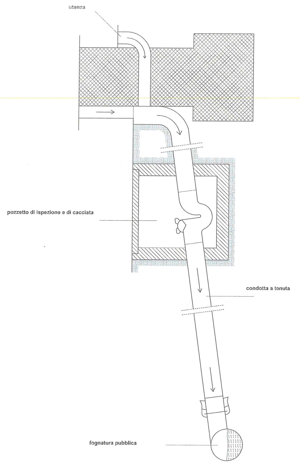
particolare pozzetto di ispezione e di cacciata, scala 1:10
